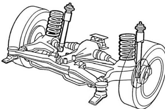
Eje trasero con suspensión de brazo semitirado.
